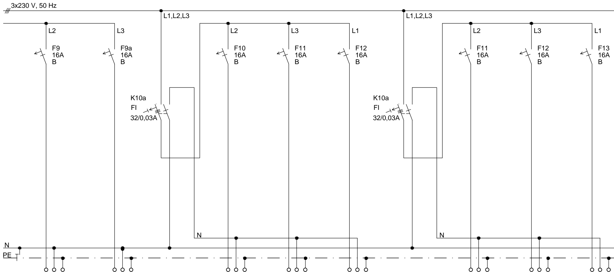
Elektromedikai hálózat
